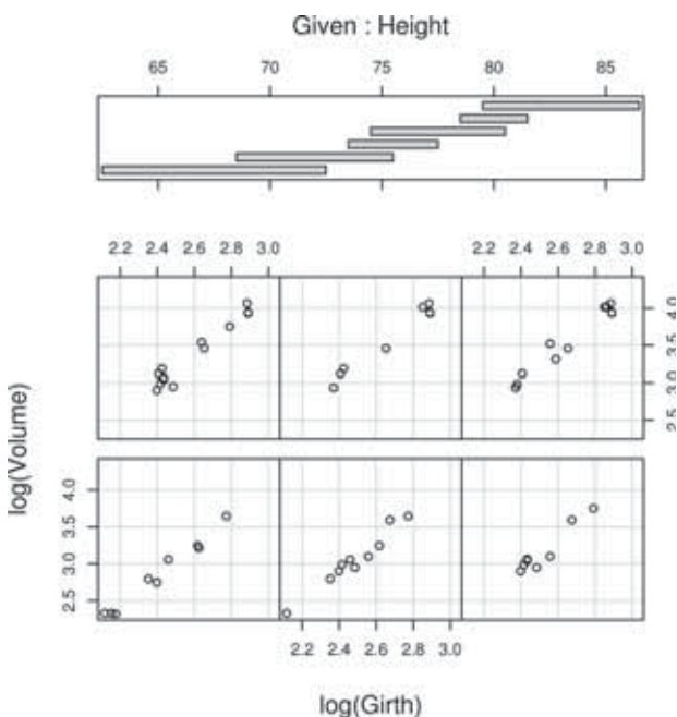
► Рис. 4. График-решетка.
