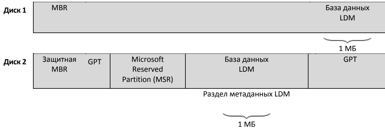
Динамический MBR-диск (Диск 1) и динамический GPT-диск (Диск 2).
