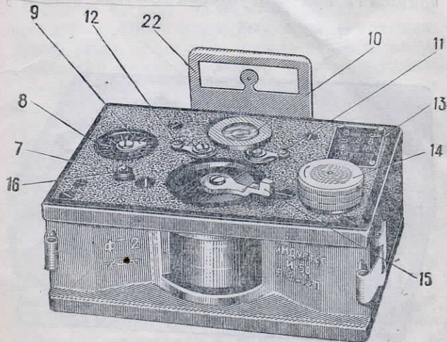
Рис. 2. Общий вид фотокамеры ФТ-2.
