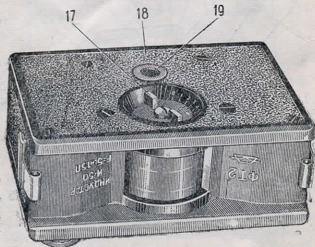
Рис. 3. Фотосамера ФТ-2. Вид на нижнюю крышку.
