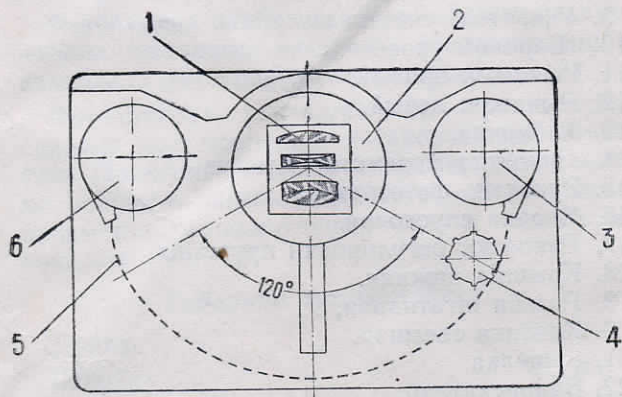
Рис. 1. Схема фотокамеры ФТ-2.
