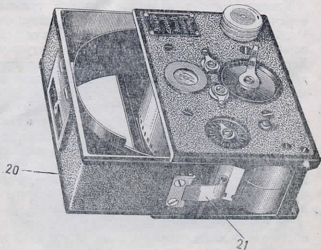
Рис. 4. Фотокамера ФТ-2. Вид на боковые стенки.
