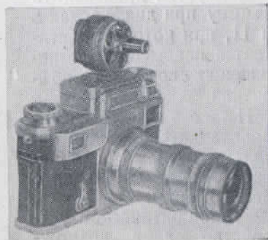
Рис. 23. Аппарат с универсальным видоискателем.
