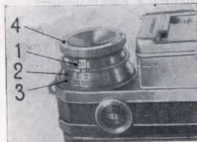
Рис. 34. Головка обратной перемотки мод. III.
