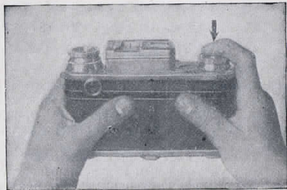
Рис. 35. Спуск затвора.
