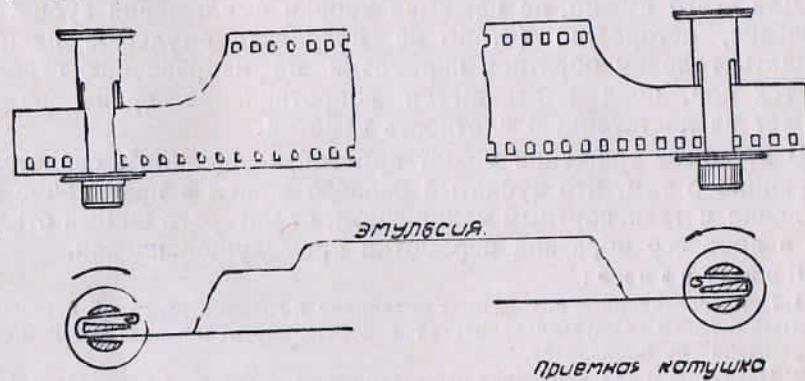
Рис. 7. Схема заправки пленки.
