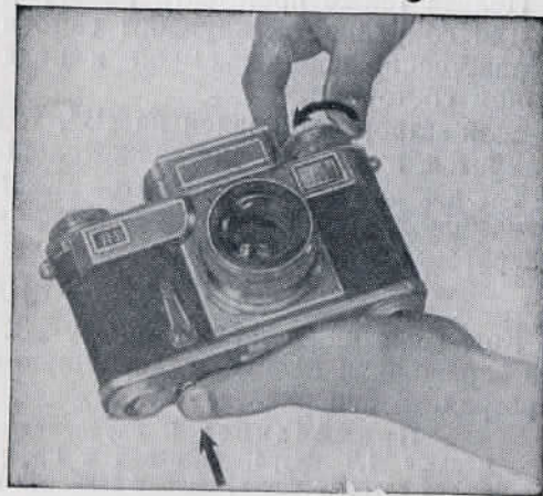
Рис. 27. Обратная перемотка.
