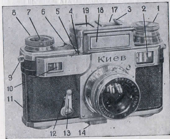
Рис. 31. Общий вид фотоаппарата „Киев“-III.
