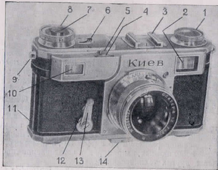
Рис. 1. Общий вид фотоаппарата „Киев“-II.
