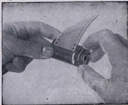
Рис. 11. Закрывание кассеты.
