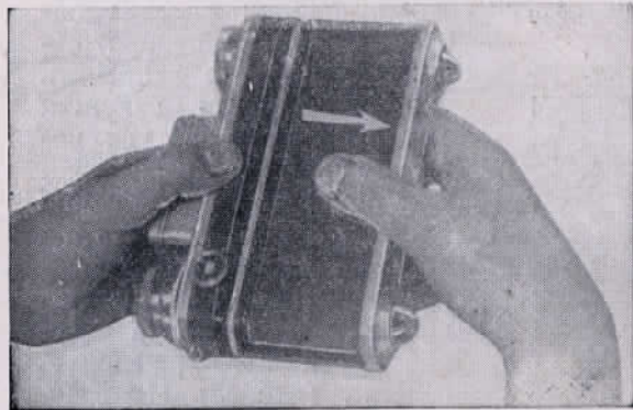
Рис. 4. Снятие задней крышки.
