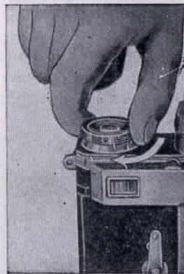
Рис. 14. Завод аппарата.
