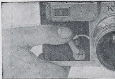
Рис. 25. Взвод рычага самоспуска.
