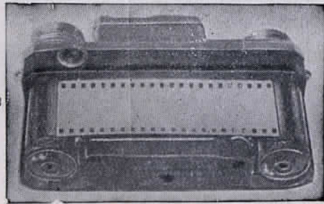
Рис. 16. Аппарат заряжен двумя кассетами.
