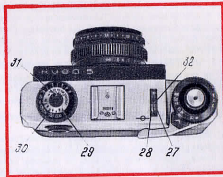
Рис. 19. Устройство экспонометра:
