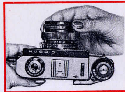
Рис. 13. Диафрагмирование объектива
