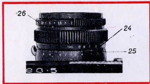
Рис. 3. Объектив «Юпитер-8НБ»:
