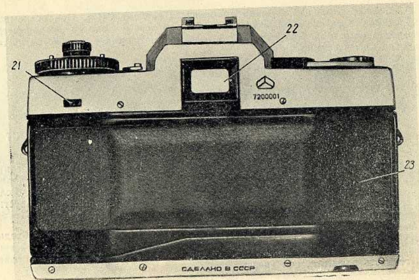
Рис. 4. Вид фотоаппарата сзади: 21—окно контроля движения пленки; 22—окуляр видоискателя; 23—откидная задняя стенка.
