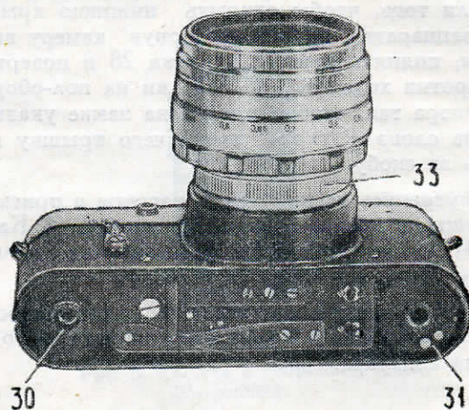
Рис. 4. Фотоаппарат «Зенит-3» (с открытой нижней крышкой) 30—катушка, 31—кассета, 33—накатка корпуса объектива.
