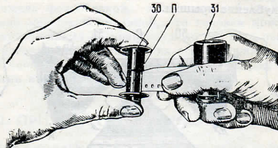
Рис. 8. Порядок крепления фотопленки на приемной катушке 30—приемная катушка, «П»—пружина, 31—кассета.
