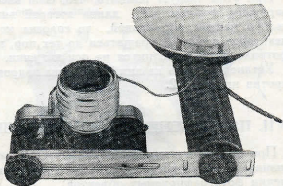
Рис. 10. Закрепление осветительного устройства на нижней крышке фотоаппарата.
