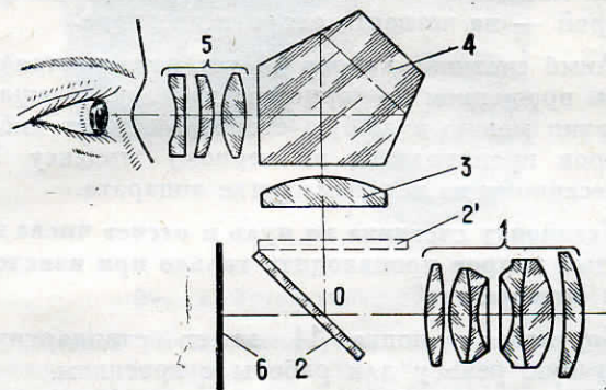
Рис. 1. Оптическая схема видоискателя
