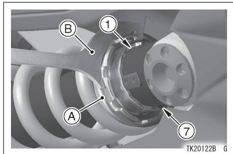
A. Регулятор предварительного поджатия пружины.
